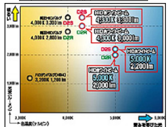
光束と色温度の相関イメージグラフ
