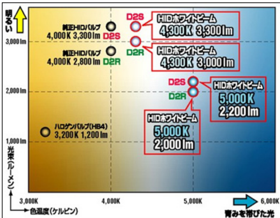
光束と色温度の相関イメージグラフ《拡大図》
