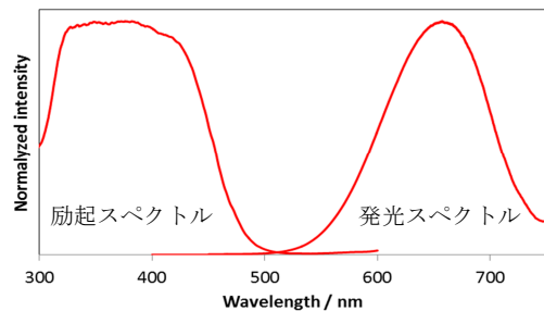
図 3. FOLP:Eu 2+ の励起-発光スペクトル
