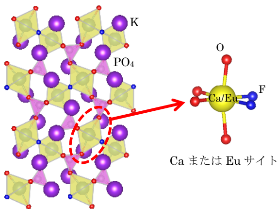
図 2. FOLP:Eu 2+ の結晶構造
